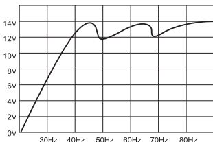
Bassleistung bei 50Hz und 70Hz ohne Pufferkondensator
