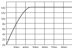
Bassleistung bei 50Hz und 70Hz mit Pufferkondensator
