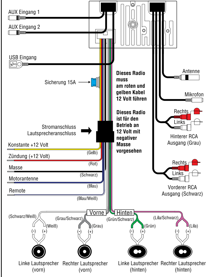
Abbildung 8 - Kabelplan
