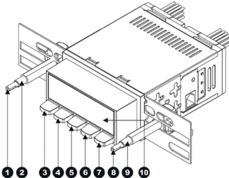
Abbildung 9 - Bedienelement
